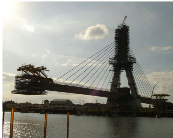
有明沿岸道路 矢部川大橋(福岡県柳川市-みやま市)
